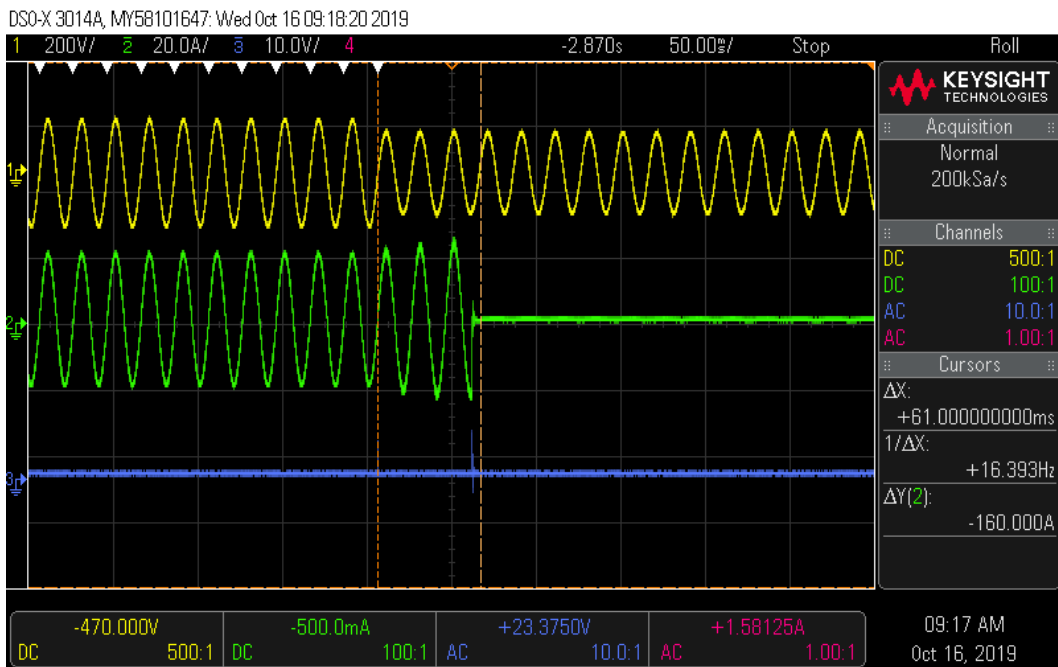
77% Un
