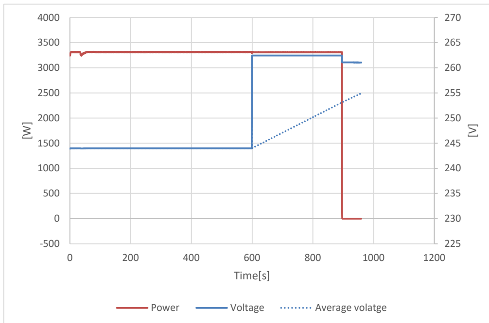
114% Un
