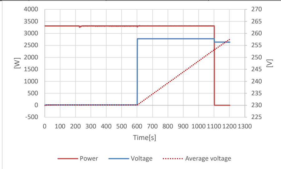
112% Un
